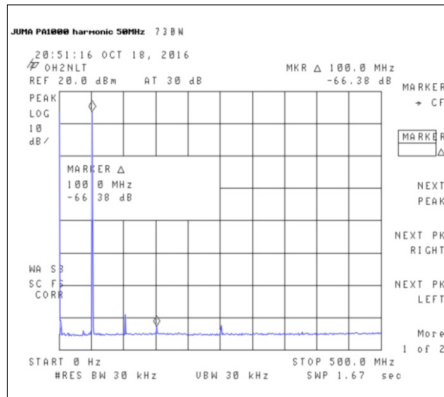
Bild 10: Nebenausstrahlungen im 6-m-Band bei Aussteuerung auf 730 W PEP Screenshot: OH2NLT
