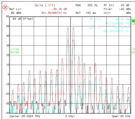
Bild 9: Intermodulation im 10-m-Band bei einer Aussteuerung auf 300 W PEP Screenshot: DL2KCK
