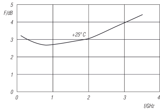
Bild 8: Rauschmaß F des SGA6489Z in Abhängigkeit von der Frequenz f bei \vartheta = 25^\circ\text{C}
