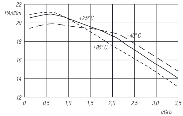
Bild 6: Ausgangsleistung P_A des SGA6489Z am 1-dB-Kompressionspunkt in Abhängigkeit von der Frequenz f bei unterschiedlichen Temperaturen
