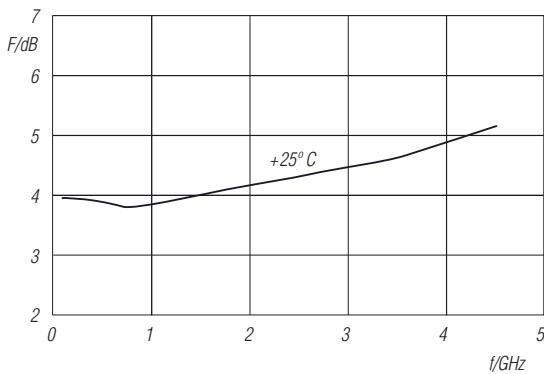
Bild 5: Rauschmaß F des SGA6289Z in Abhängigkeit von der Frequenz f bei \vartheta = 25^\circ\text{C}
