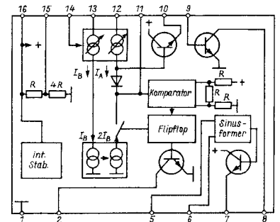
Bild 1: Prinzipienschaltung
