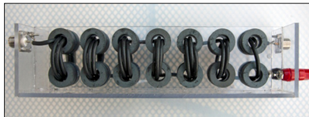
Bild A3: Seite zwei des Kellermann-Baluns mit FRK-25-N30
