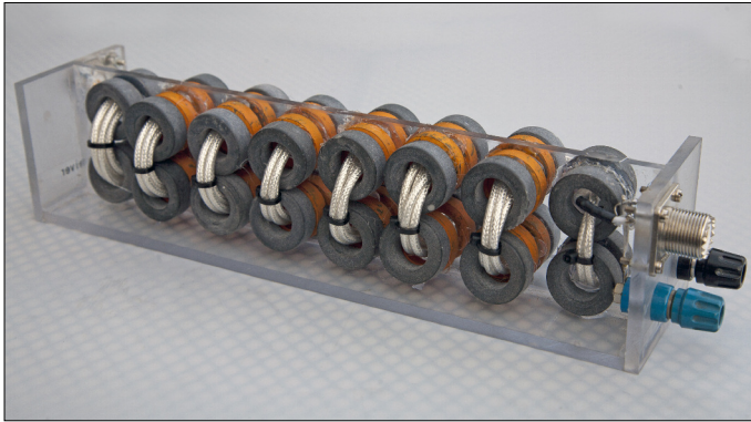
Bild A1: Kellermann-Balun, hier gemischte Bestückung aus FRK-25-N30 und K3/1200
