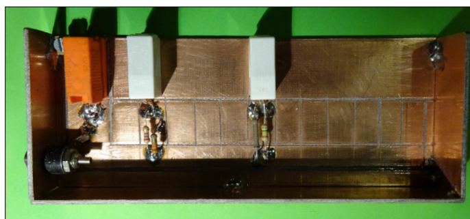
Ansicht der nahezu vollständig bestückten Leiterplatte
