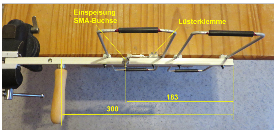
Bild 15: Die Einspeisung in Seitenansicht
